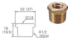
変換アダプター 576-232 ¥380 (税込 ¥399) 1/- 576-233 ¥640 (税込 ¥672) 1/-
