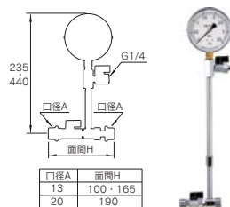
水道メーター用水圧テスター (Gネジ用) 6498G ¥19,800 (税込 ¥20,790) 1/5
