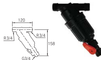
Y型ストレーナー (コックつき) 20 5759 ¥6,900 (税込 ¥7,245) 1/- 575-901 ¥7,300 (税込 ¥7,665) 1/-
